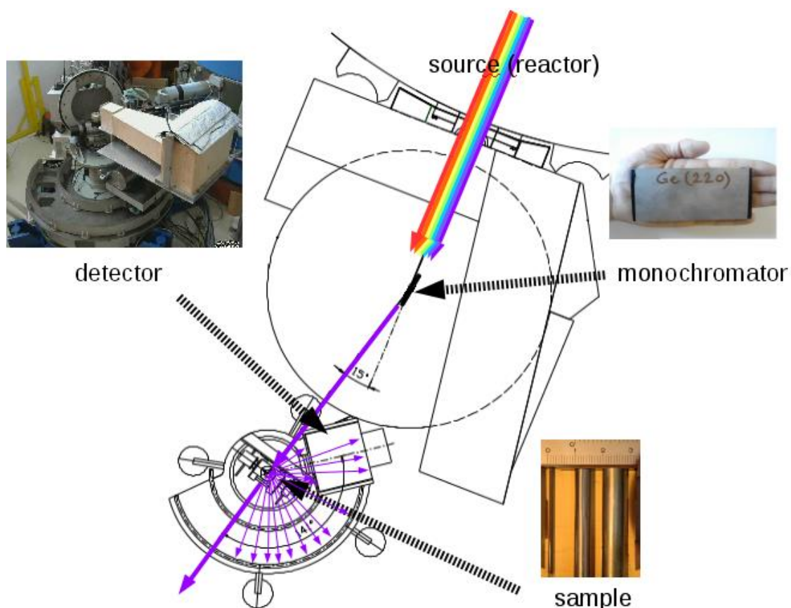
Figure 2. Overview of the MTEST ver 3.0 diffractometer (Modified from ver 2.0 layout, whose source: L. Temleitner, L. Pusztai, Sz. Pothoczki: Tetraéderes molekuláris folyadékok – Egyszerű anyagok, fejfájást okozó problémák [in Hungarian: The structure of neat liquids consisting of tetrahedral molecules – Simple materials that have caused a lot of headache], Természet Világa, 147 (2016,8) 346.)
